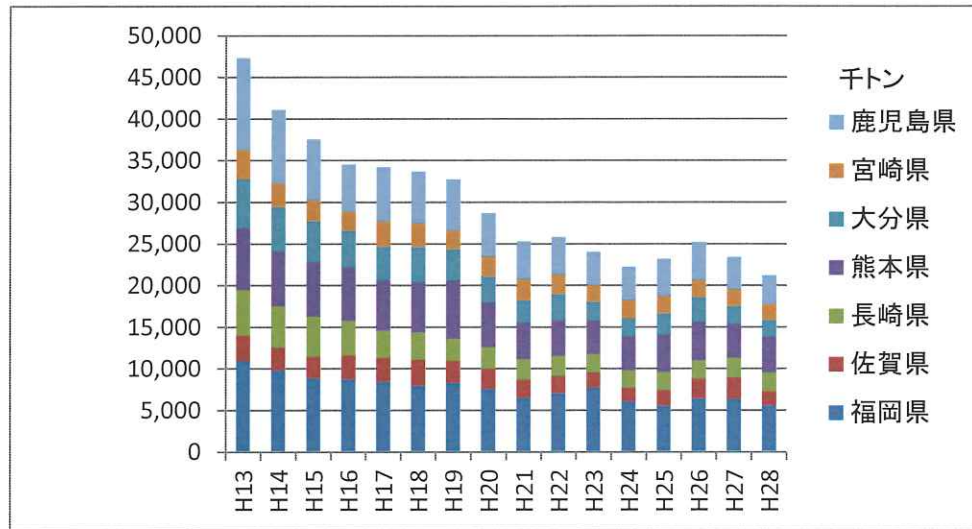
九州各県の生産量(砕骨材)
