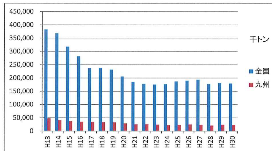
全国及び九州の生産量(砕骨材)
